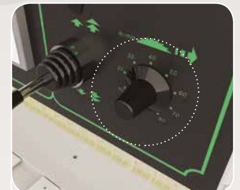
Avanzamento lama con variatore di velocità 0-80 mt/min Blade feed with precision speed variator 0-80 round / min Avancement de la lame avec variateur de vitesse 0-80 mt / min Avance de la hoja con variador de velocidad 0-80 mt / min
